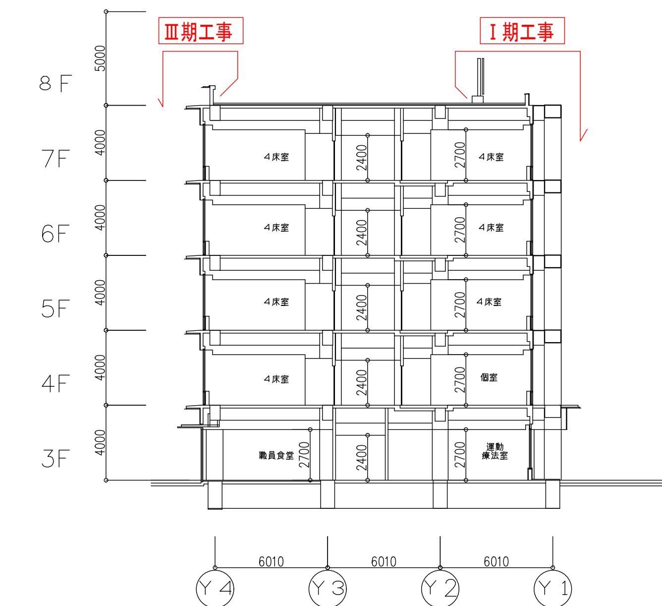
×9-×10通り断面図
