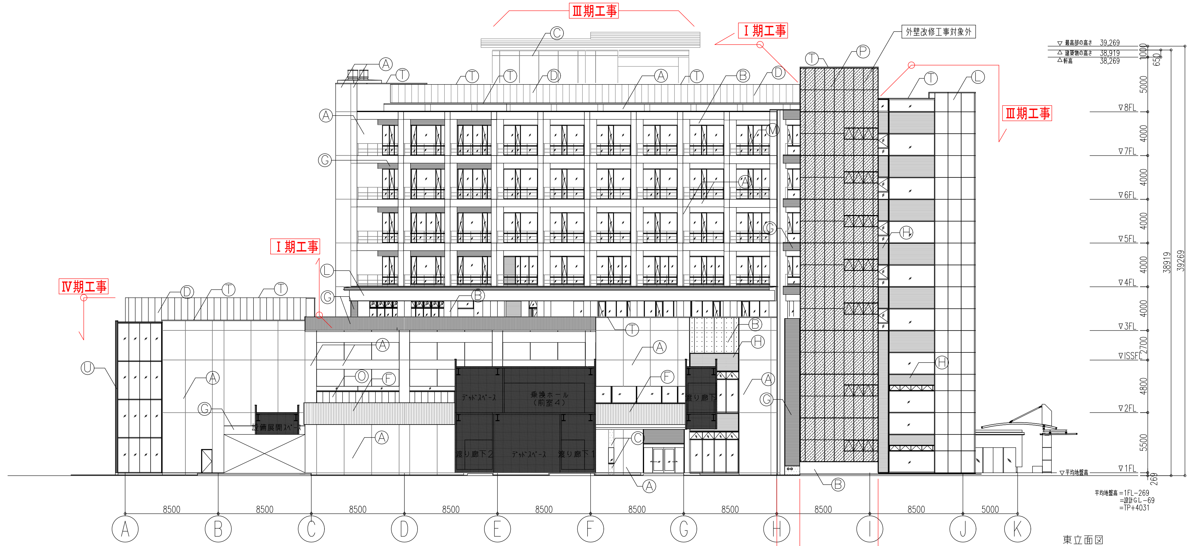
東立面図
