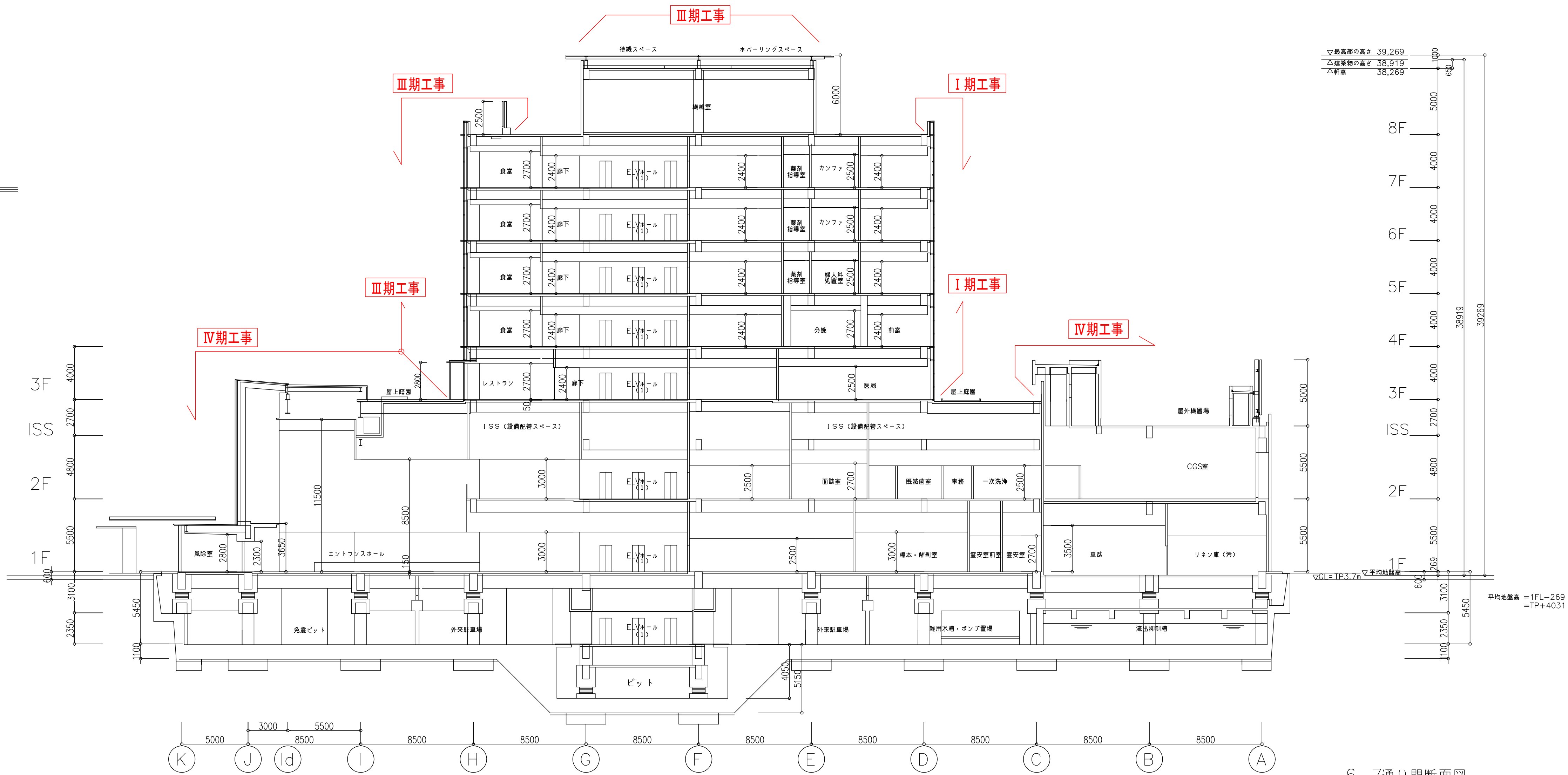
6-7通り断面図
