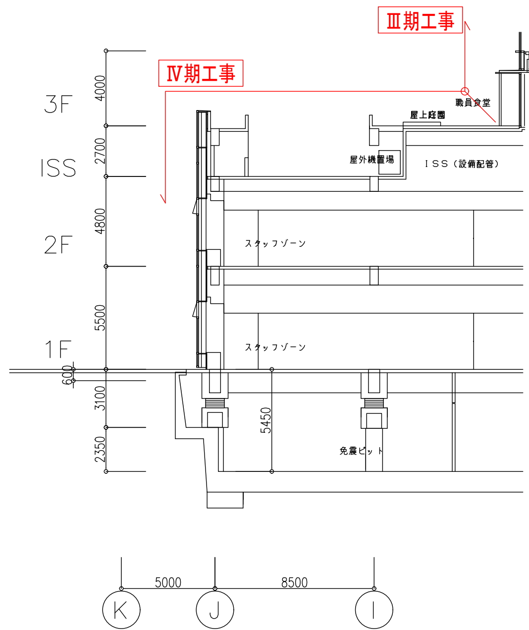
9-10通り断面図
