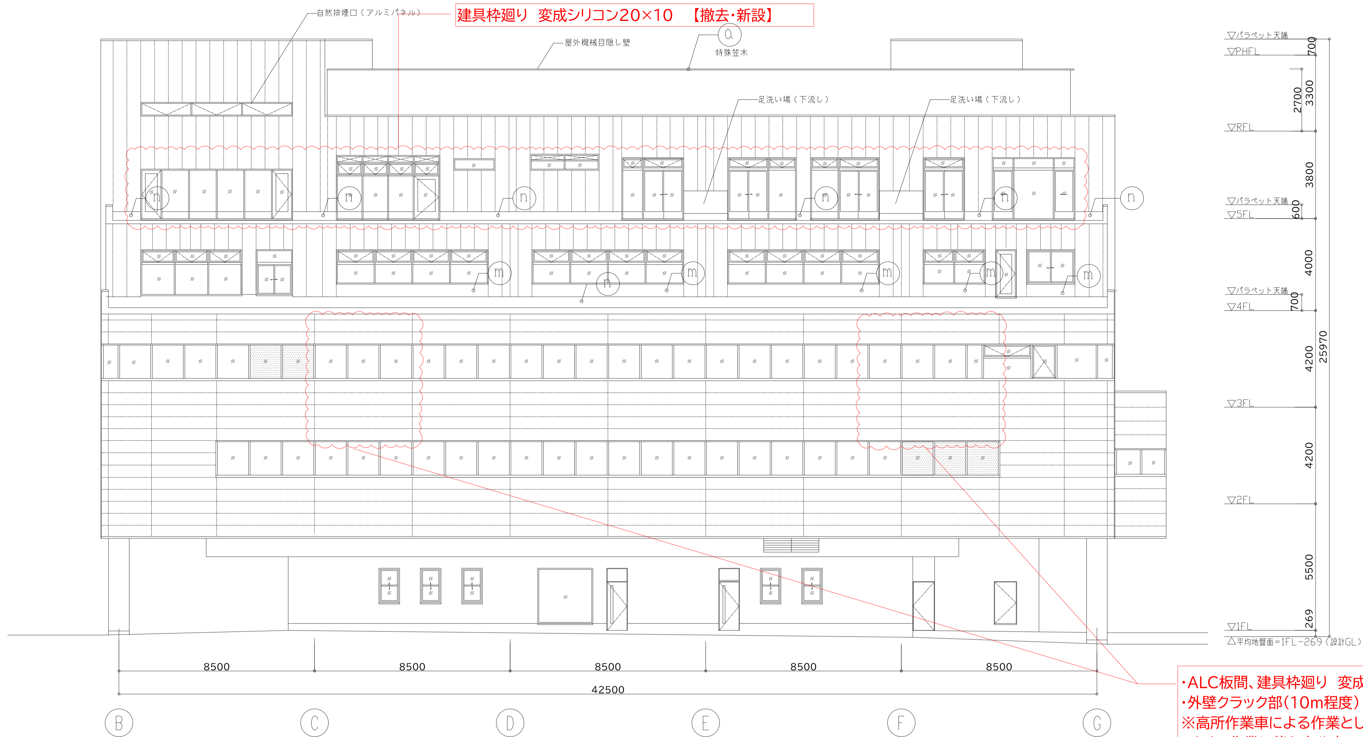
東側立面図 (NS)
